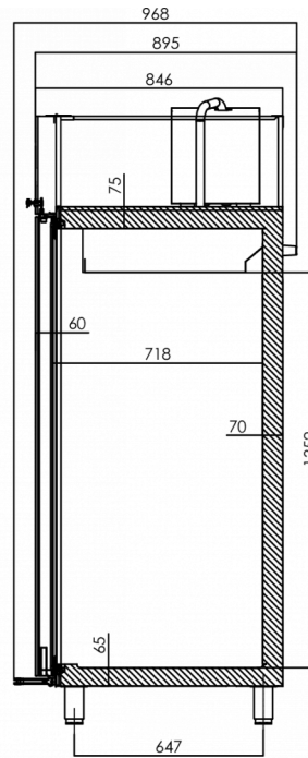
SECTION A-A
